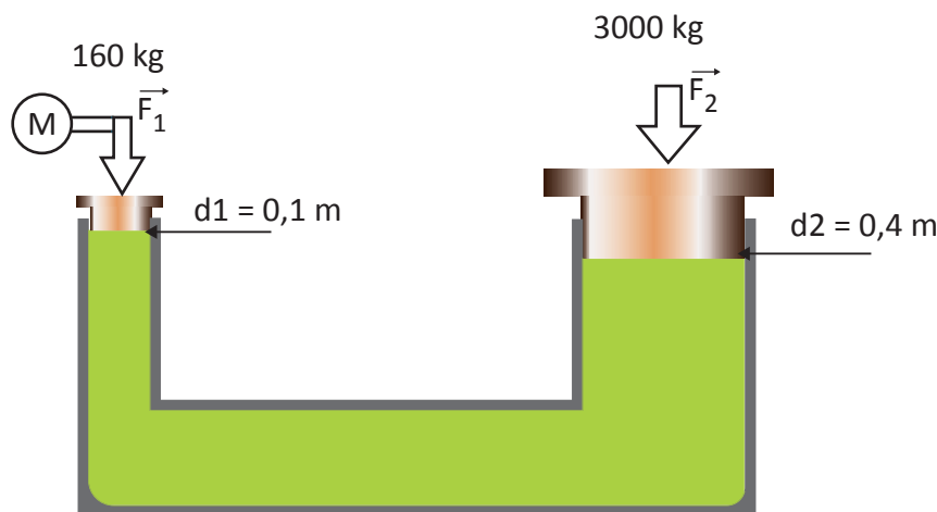
Figura: esquema de elevador hidráulico.
